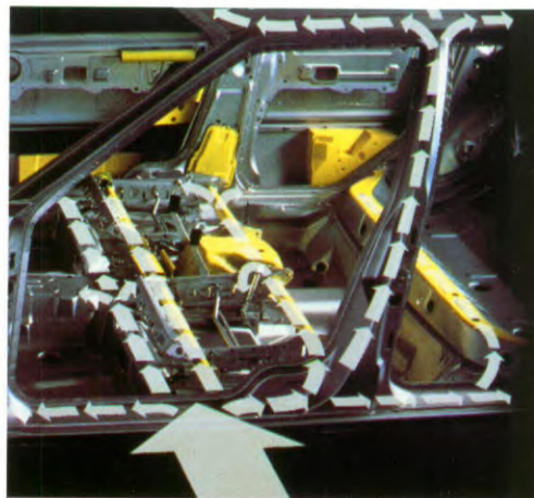
SIPS, het Side Impact Protection System van Volvo, zorgt ervoor dat de krachten die vrijkomen bij een botsing geabsorbeerd en verspreid worden via dwarsprofielen, stijlen, de vloer, het dak en andere onderdelen van de carrosserie. Hierdoor kan een Volvo een zijdelingse botsing veel beter 'opvangen' dan auto's met een conventioneel beschermingssysteem.
