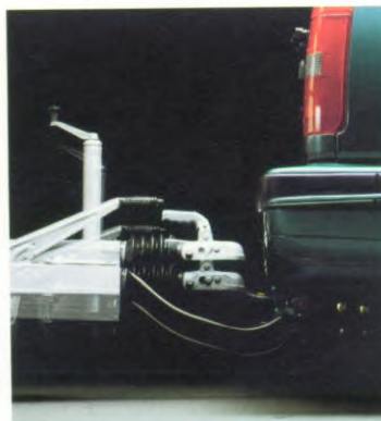
❑ Automatische niveauregeling
