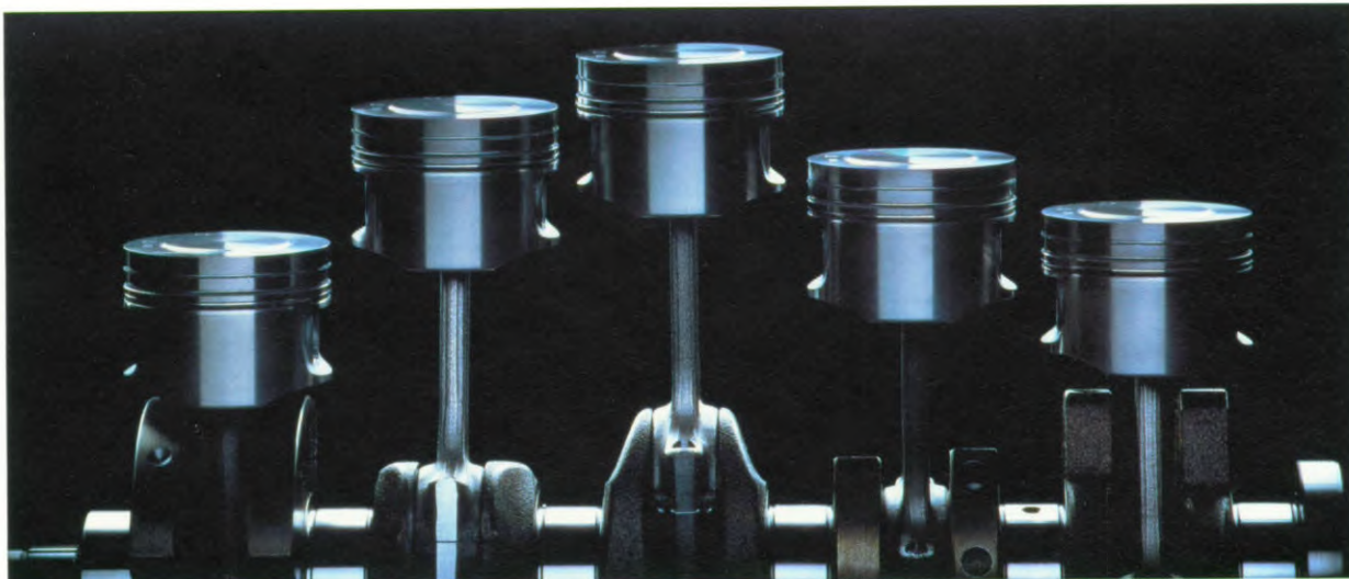
De dwarsgeplaatste vijfcilinder krachtbron heeft de trekkracht en souplesse van een zescilindermotor... maar daarbij is de motorruimte niet groter of de passagiersruimte niet kleiner.
